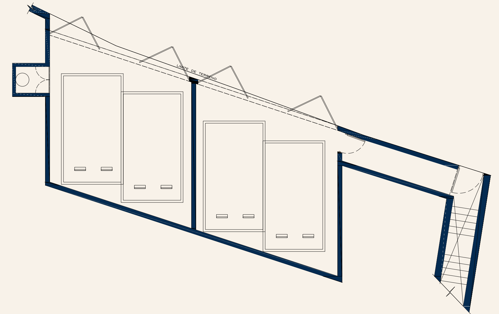
PLANTA ESTACIONAMIENTO
