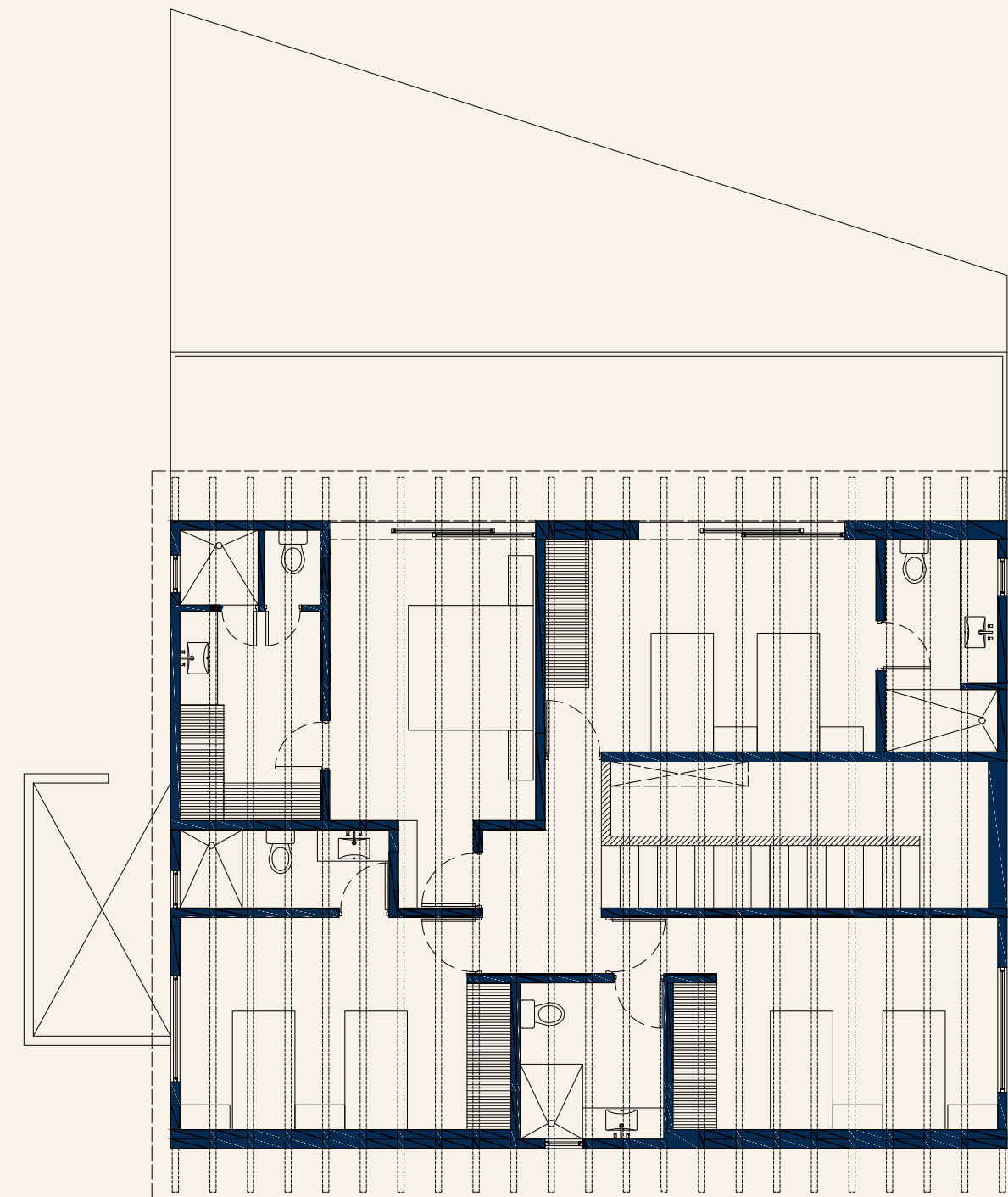
PLANTA ALTA
